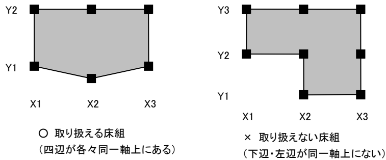
図 3.1.2-5 取り扱える床組形状
