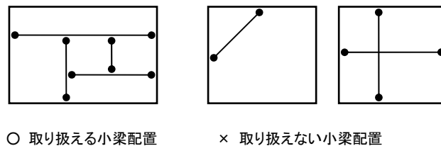
図 3.1.2-6 取り扱える小梁配置
