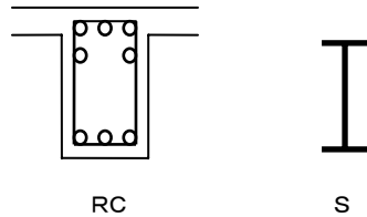
図 3.1.2-2 大梁の断面形状
