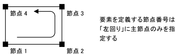
図 6-2-10 要素の定義方法
