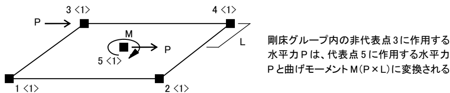
図4-1-7 剛床グループの非代表節点に作用する水平力
