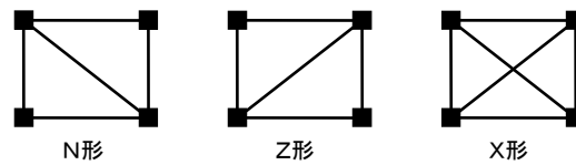
図 3-3-14 斜め材の形状
