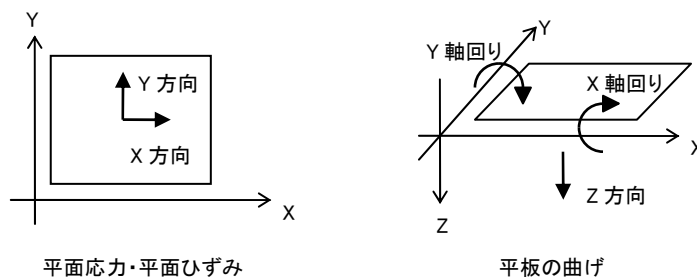
図 6-1-4 自由度
