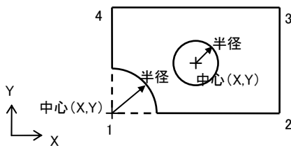
図 6-2-3 穴の指定方法
