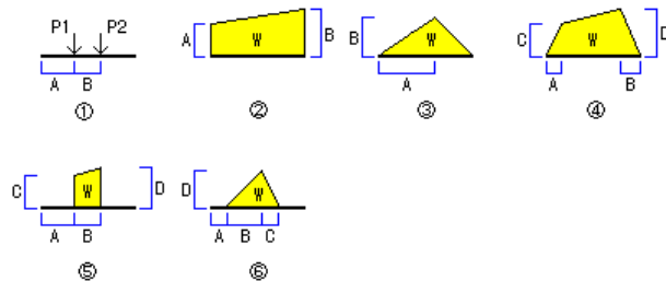
図 3-3-8 荷重形一覧
