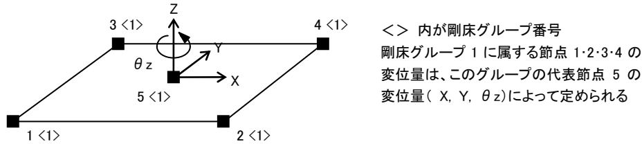
図4-1-6 剛床グループと代表節点
