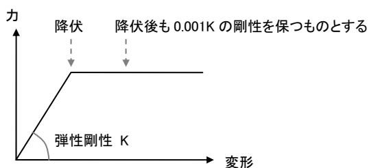
図 3-1-2 バイリニア型の弾塑性特性
