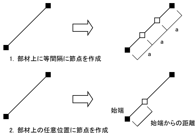
図 4-3-3 部材の分割
