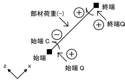
図 4-3-2 荷重項の符号
