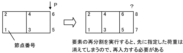
図 6-2-4 要素の再分割後の節点荷重
