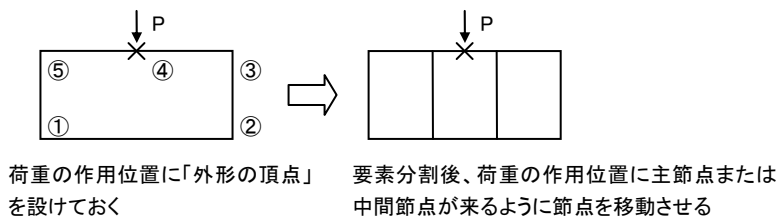
図 6-2-6 外形線分の中間に作用する集中荷重
