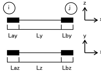
図 9-1-2 剛域をもつ部材
