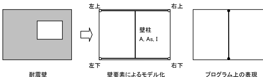
図 3-1-7 壁要素
