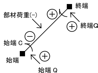
図 3-3-5 荷重項の符号
