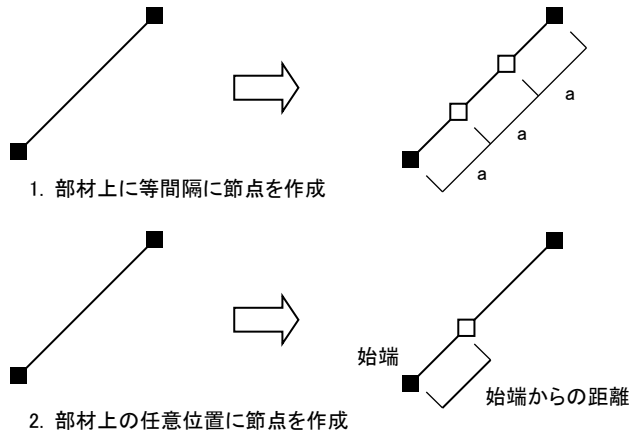
図 3-3-6 部材の分割
