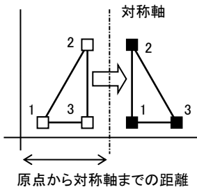
図 3-3-11 反転
