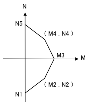
図 3-3-1 M-N 耐力線
