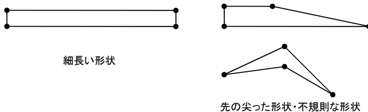
図 6-1-10 好ましくない要素形状
